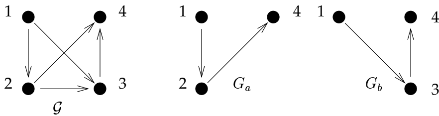
Abbildung 4.1: Graph \mathcal{G} aus Satz 55, sowie die im Beweis auftretenden Subgraphen
