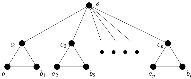
Abbildung 4.2: Der Graph G aus dem Beweis von Satz 57
